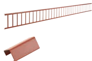
Griglia fermaneve piena 3 m di lunghezza incl. morsetti di collegamento Codice ordine funzione 4070
