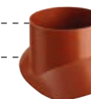
Adattatore uscita termica sistema 70/110, inclinazione del tetto 20°-50°, tenuta al calore max. 60°C Codice ordine funzione 3086
